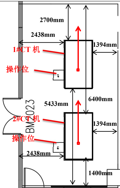
图 1-4 2#CT 室平面布置图
