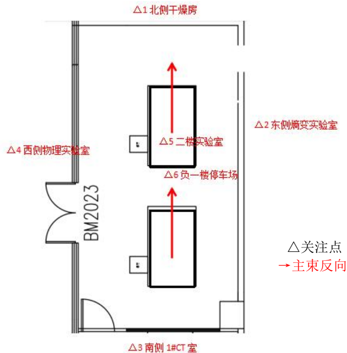
图 11-1 工业 CT 机的摆放位置图
