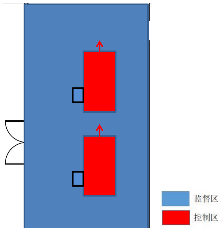
图 1-5 CT 机控制区和监督区图
