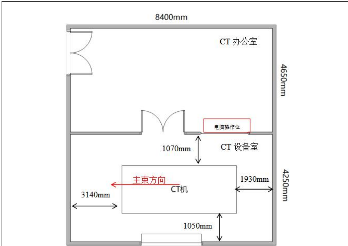
图 1-4 CT 检测室平面布置图
