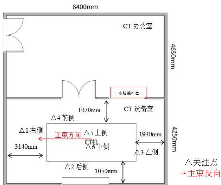
图 11-1 工业 CT 机的摆放位置图
