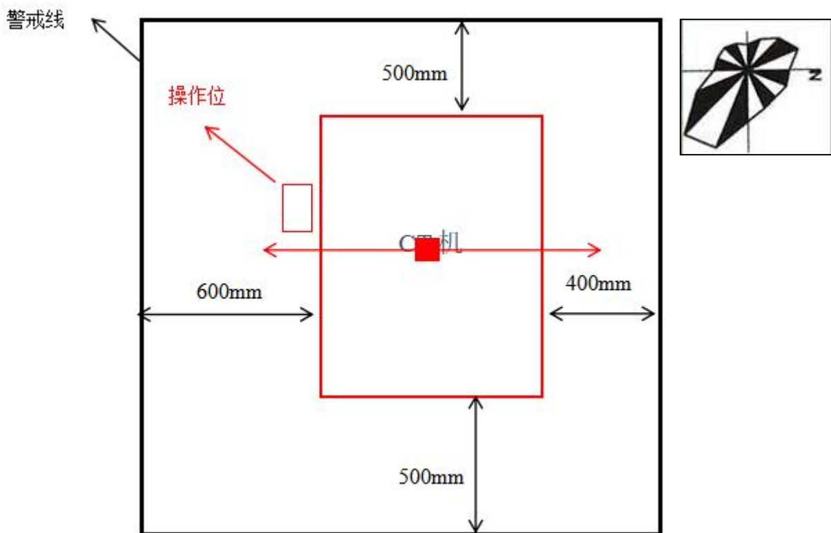
图 1.3-3 储能工厂 2#CT 检测区平面布置图
