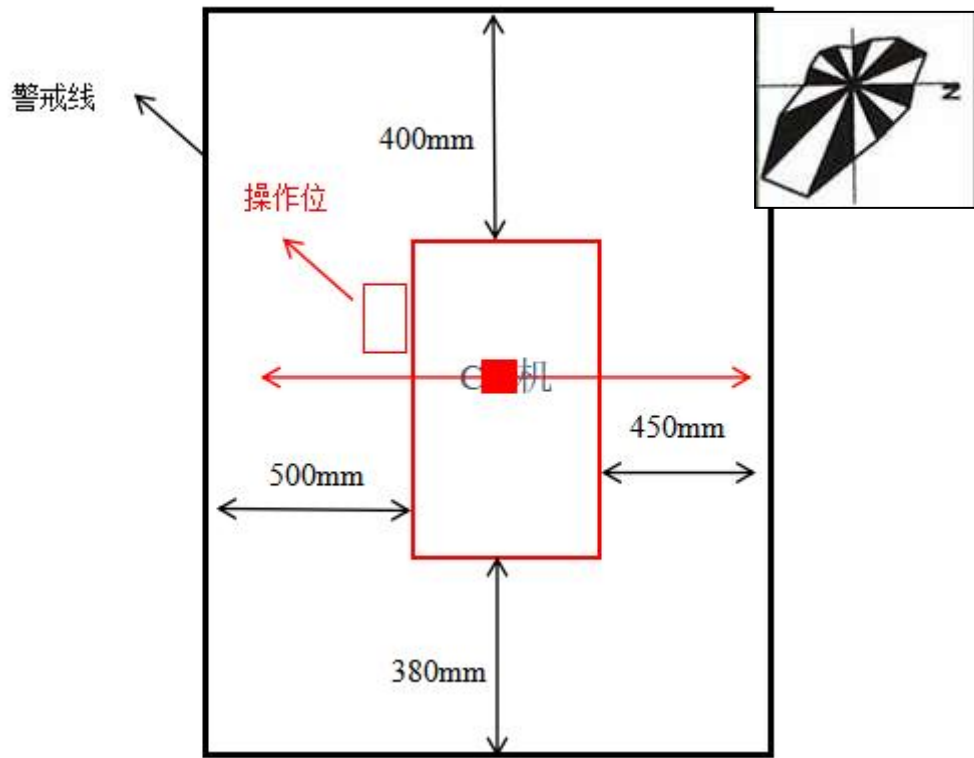
图 1.3-3.1 储能工厂 1#CT 检测区平面布置图
