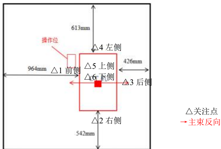
图 11-2 工程中心 CT 机的摆放位置图
