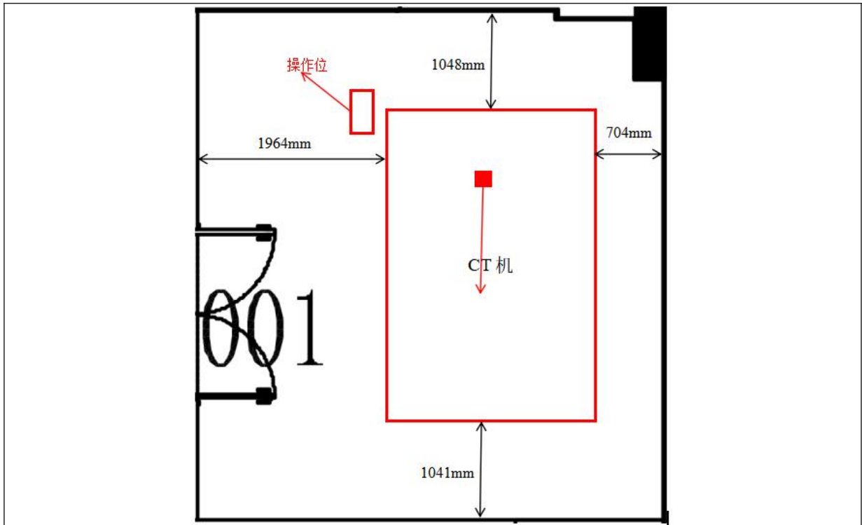
图 1.1-4 创新实验室 CT 室平面布置图
