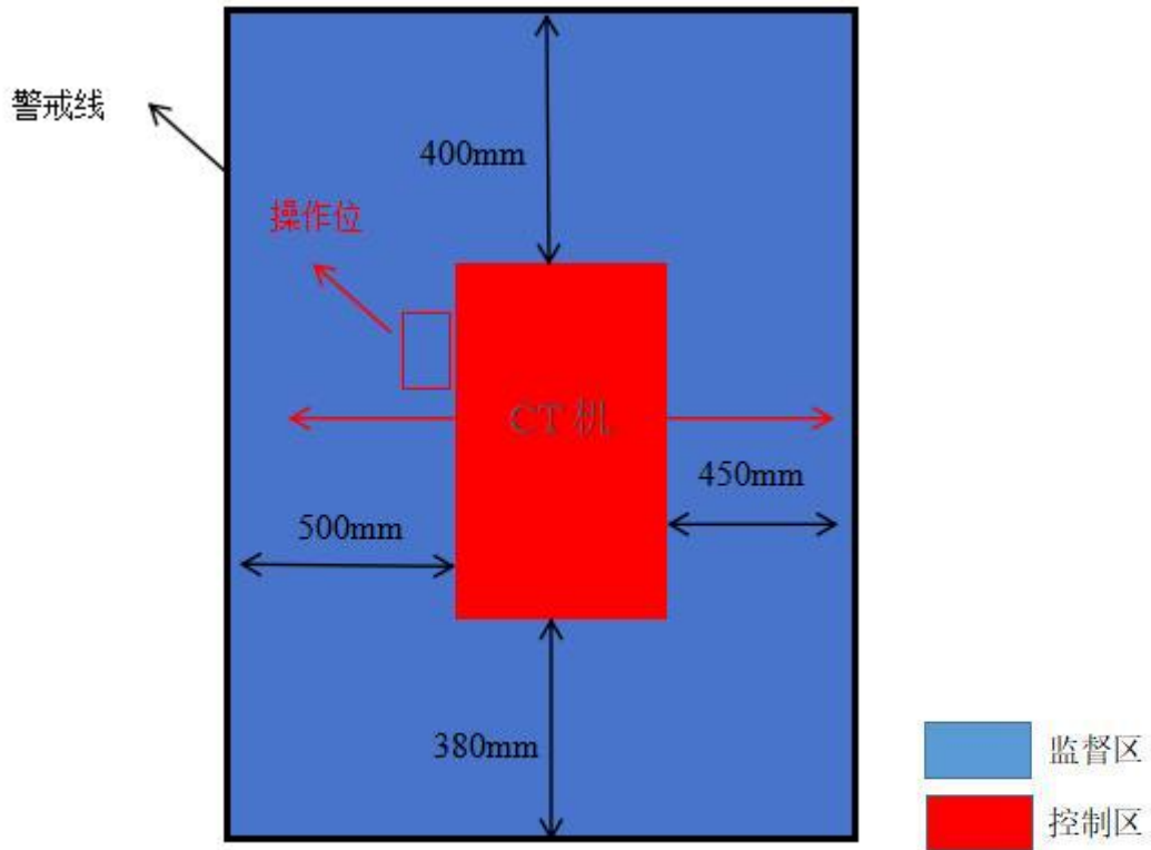
图 1.3-4.1 储能工厂 1#CT 检测区控制区和监督区图
