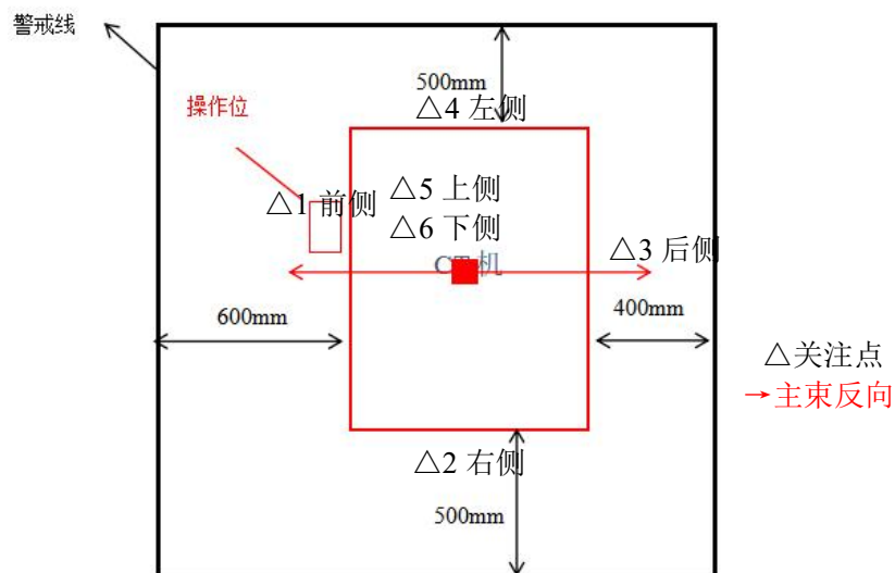
图 11-4 储能工厂 2#CT 机的摆放位置图
