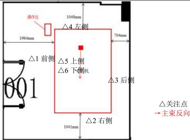
图 11-1 创新实验室 CT 机的摆放位置图
