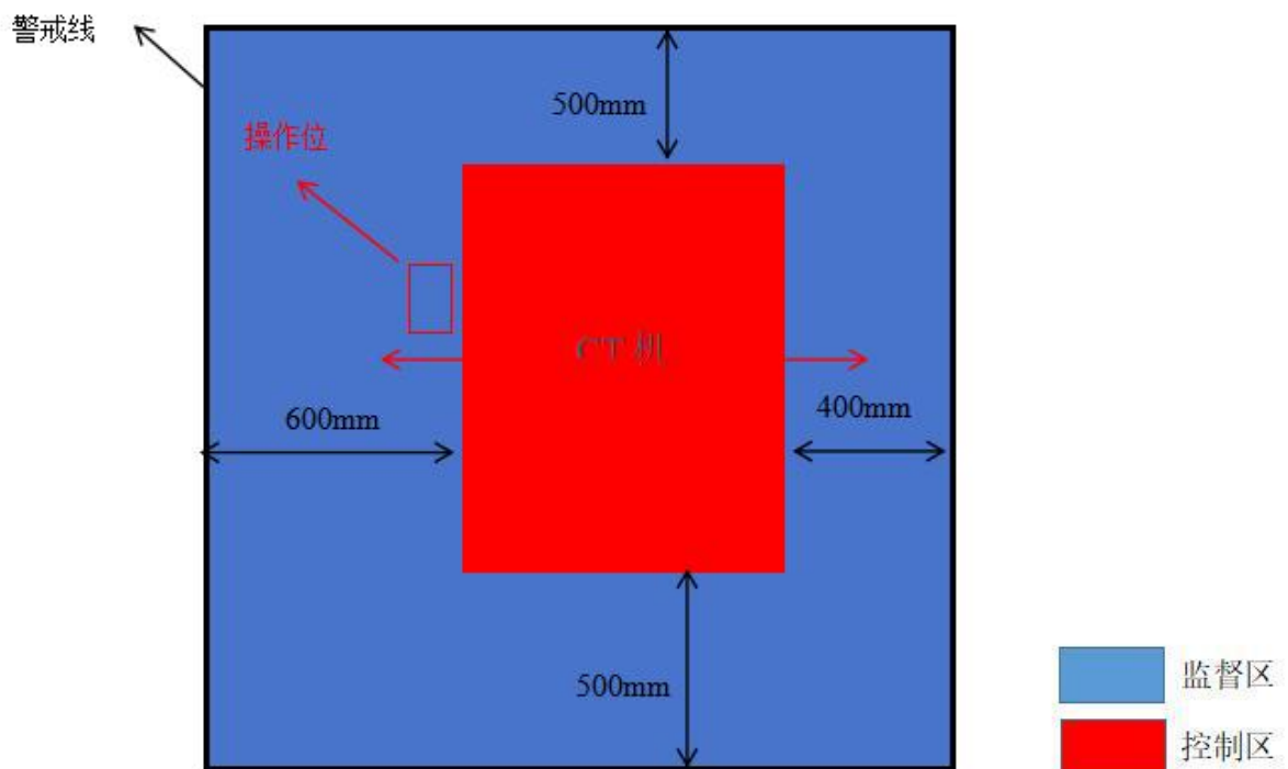
图 1.3-4.2 储能工厂 2#CT 检测区控制区和监督区图
