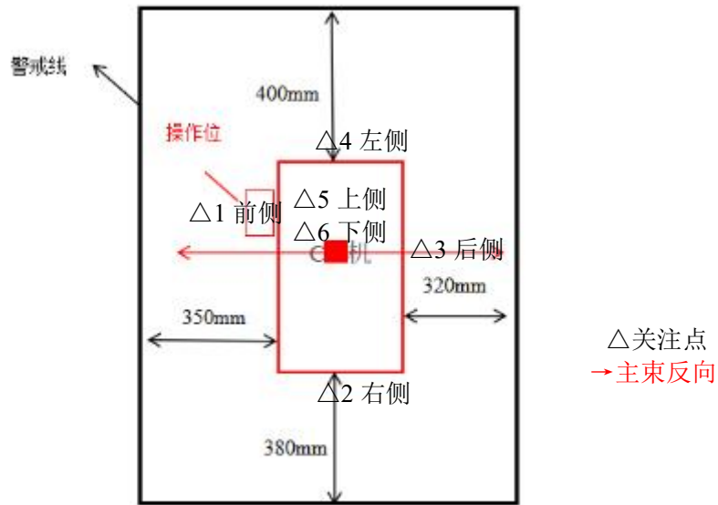
图 11-3 储能工厂 1#CT 机的摆放位置图
