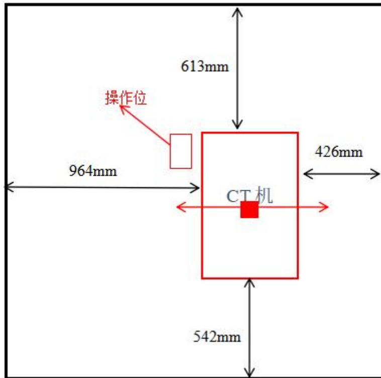
图 1.2-3 工程中心 CT 检测区平面布置图
