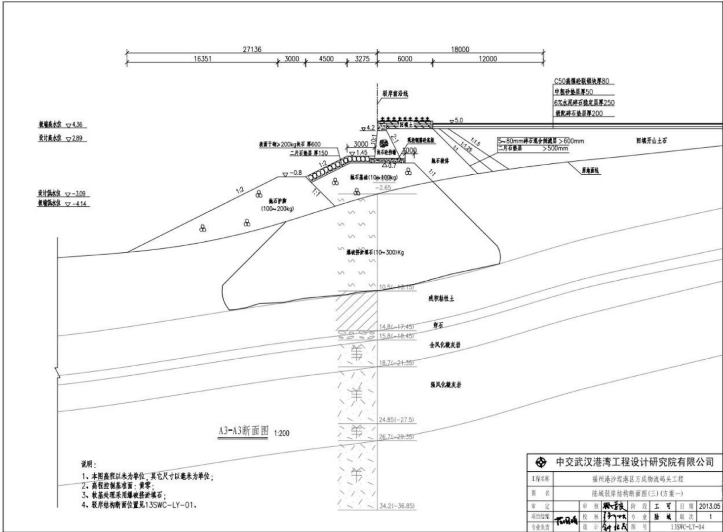
图 2.5-4 项目陆域驳岸结构断面图（3）
