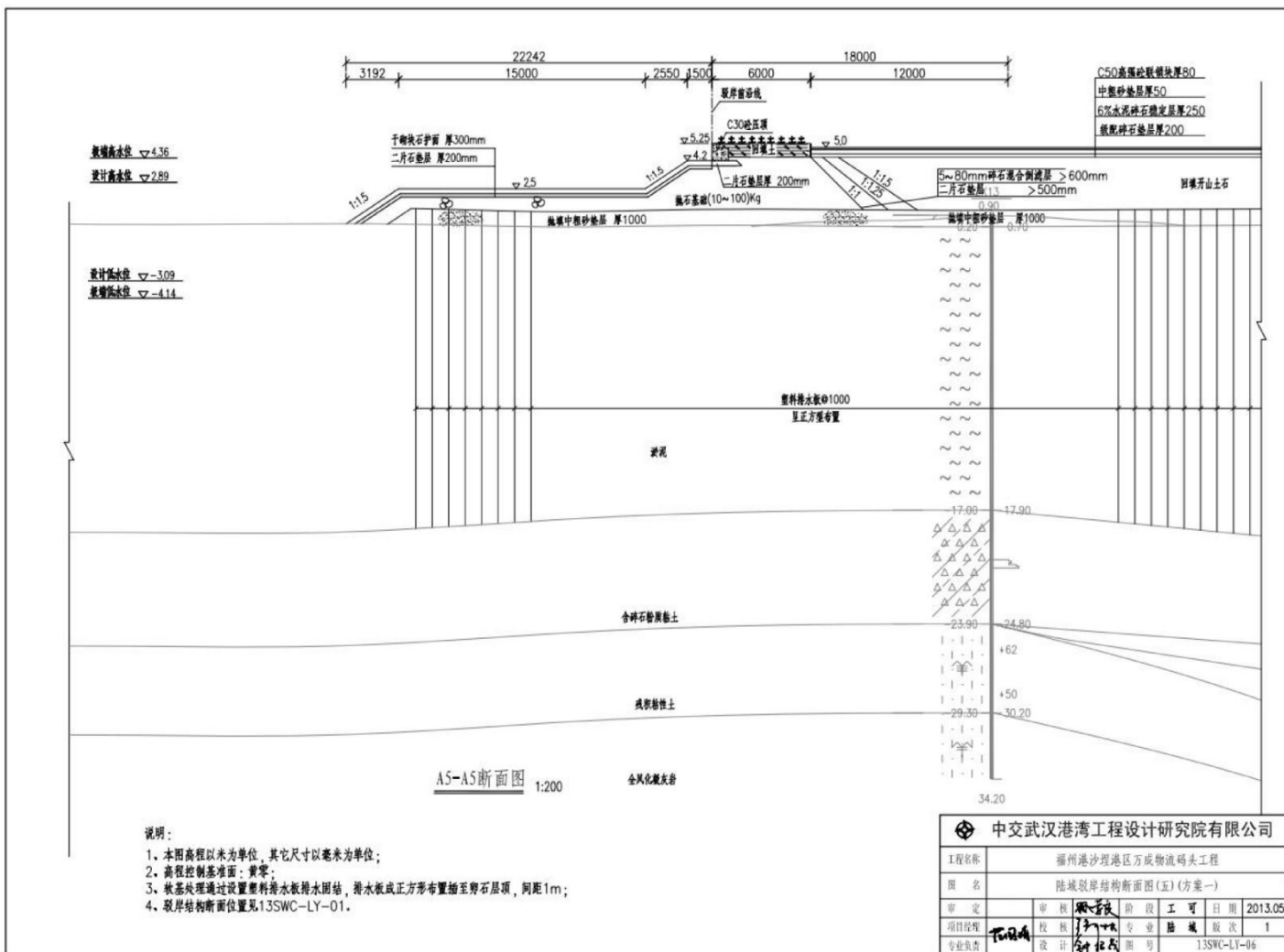
图 2.5-6 项目陆域驳岸结构断面图 (5)
